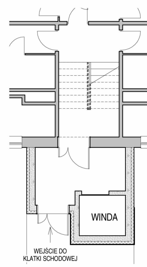
RZUT SKALA 1:100
